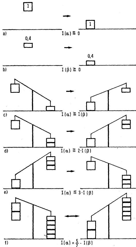
Abb. 2: Irreversibilitätsvergleich für zwei Prozesse der Art »(Verbrauch) von mechanischer Energie«.
