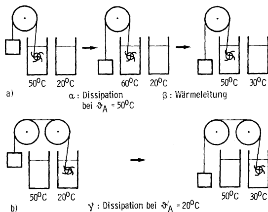
Abb. 4: Zur Temperaturabhängigkeit der Irreversibilität: \gamma stimmt in Anfangs- und Endzustand überein mit \alpha gefolgt von \beta .
